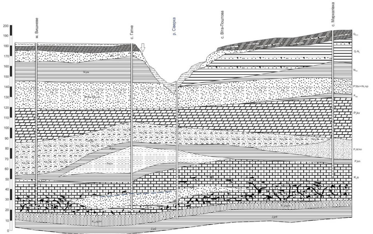
Рис. 1. Геологічний розріз по лінії I-I [3], характерний для с. Тарасівка (див. рис. 2). Fig. 1. Geological section along the line I-I [3], which is typical for Tarasivka village (see Fig. 2).
