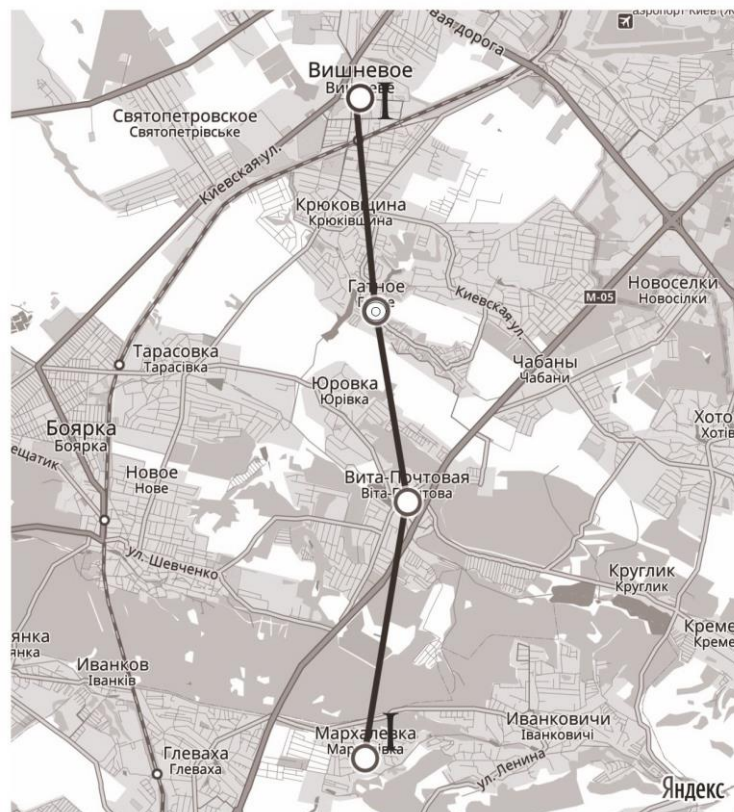
Рис. 2. Мапа району досліджень з лінією геологічного розрізу I-I. Fig. 2. Map of the research area with the line of geological section I-I.
