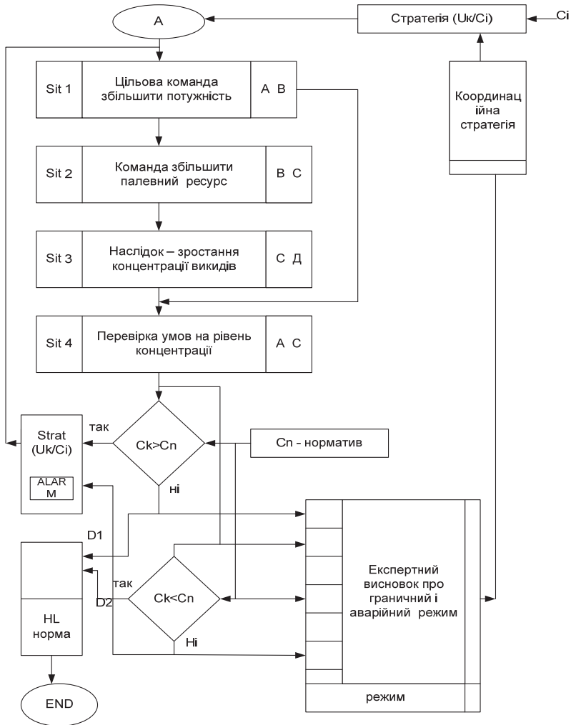
Рис. 2. Структура алгоритму побудови логічного висновку про динамічний об'єкт
