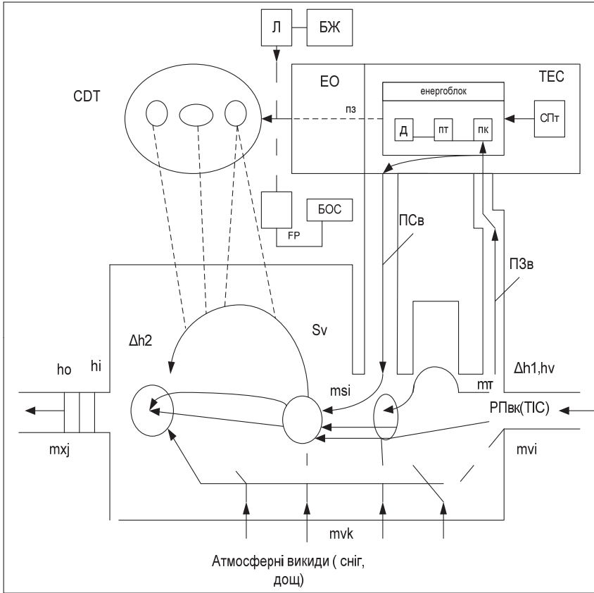
Рис. 3. Блок-схема формування потоків водних ресурсів для систем водопідготовки енергоблоків ТЭС
