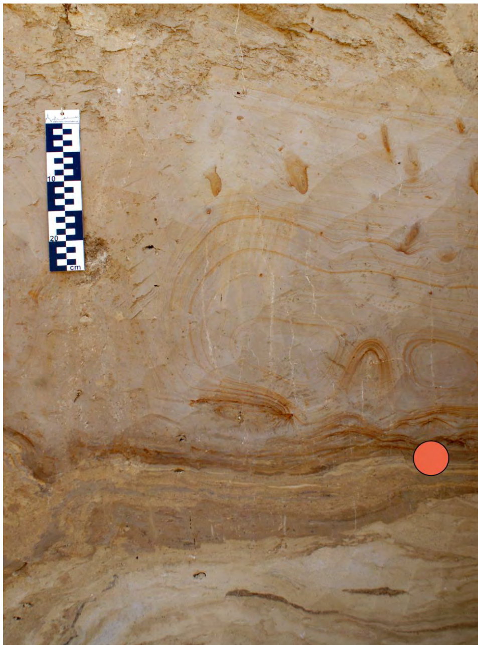
Рис. 5. Дубнівський викопний ґрунт у розрізі Чистоподи, зачистка 2021 р. (червоним колом позначено місце виявлення артефакту в 2020 р.)
