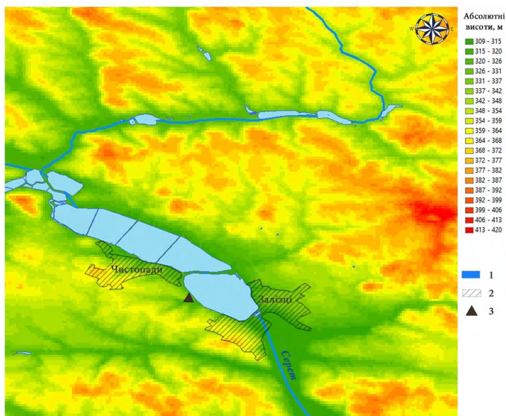
Рис. 1. Цифрова модель рельєфу околиць палеолітичної пам'ятки Чистопаді: 1 – водойми, 2 – населені пункти, 3 – палеолітична пам'ятка Чистопаді (за даними SRTM)
