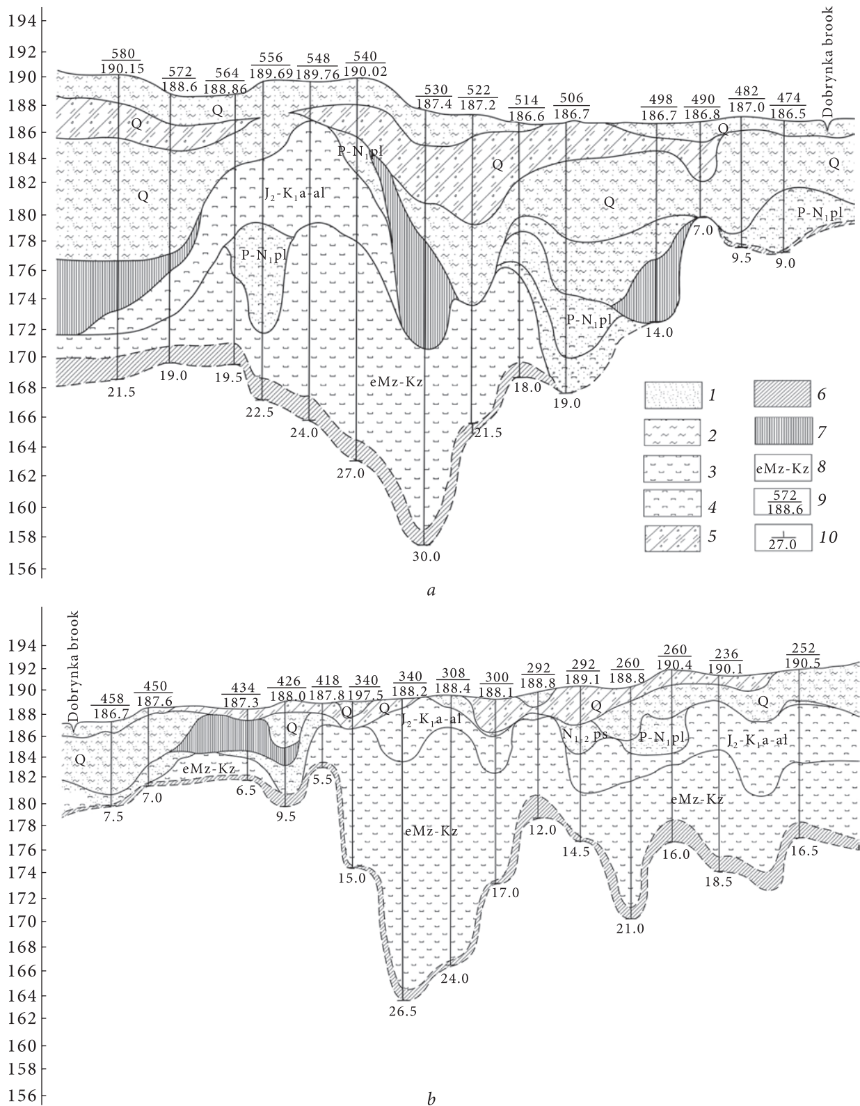
Рис. 2. Геологічні розрізи Тростяницького родовища (побудовано за даними С.К. Швайберов, 1999) (а, б): 1 — пісок; 2 — глина; 3 — каолін елювіальний; 4 — каолін флювіальний; 5 — моренні суглинки; 6 — кора вивітрювання; 7 — продуктивний горизонт; 8 — вік; 9 — номер свердловини / висота; 10 — глибина
