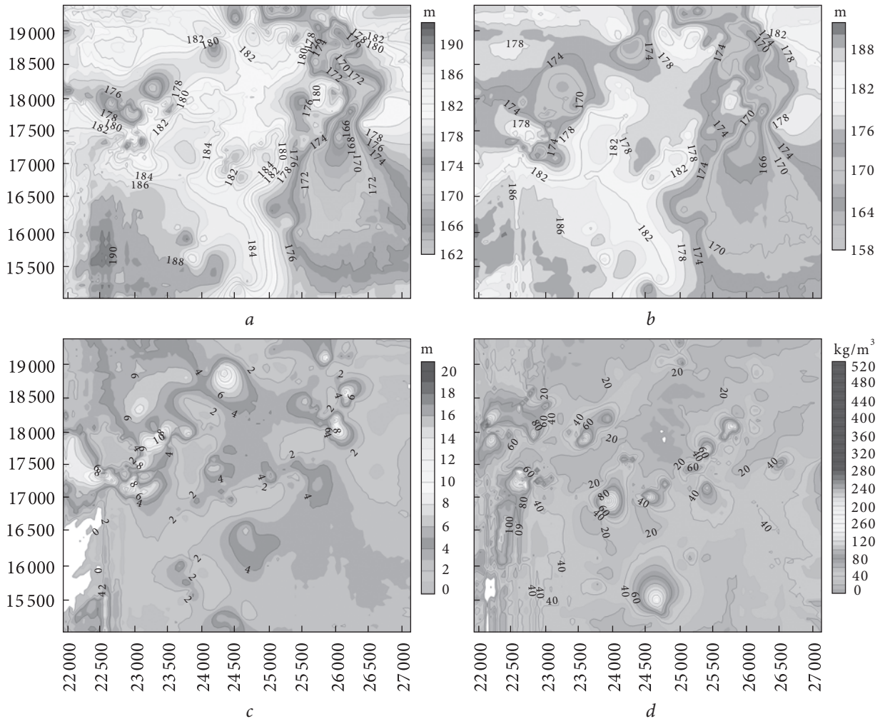
Рис. 7. Ізогіпси покрівлі (а), підшови (b), ізопакіти товщини (с) середньоярсько-нижньокрейдових алювіальних відкладів та латеральний розподіл середнього вмісту ільменіту в алювії (d). За даними детальної геологічної розвідки
