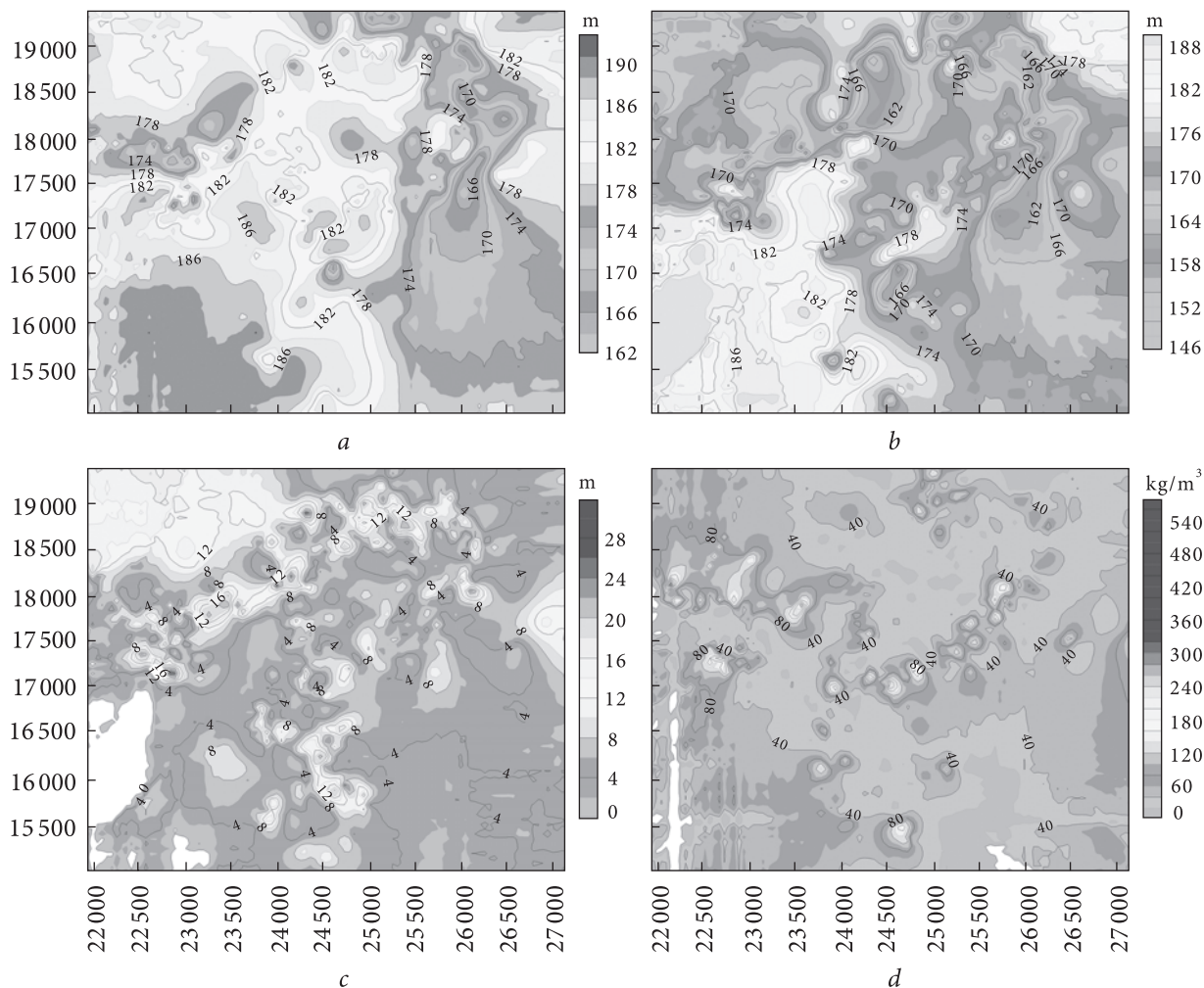
Рис. 9. Ізогіпси покрівлі (а), підшови (b), ізопакіти товщини (с) кори вивітрювання кристалічних порід фундаменту разом з середньоюрсько-нижньокрейдовими алювіальними відкладами та латеральний розподіл у цій товщі порід середнього вмісту ільменіту (d). За даними детальної геологічної розвідки
