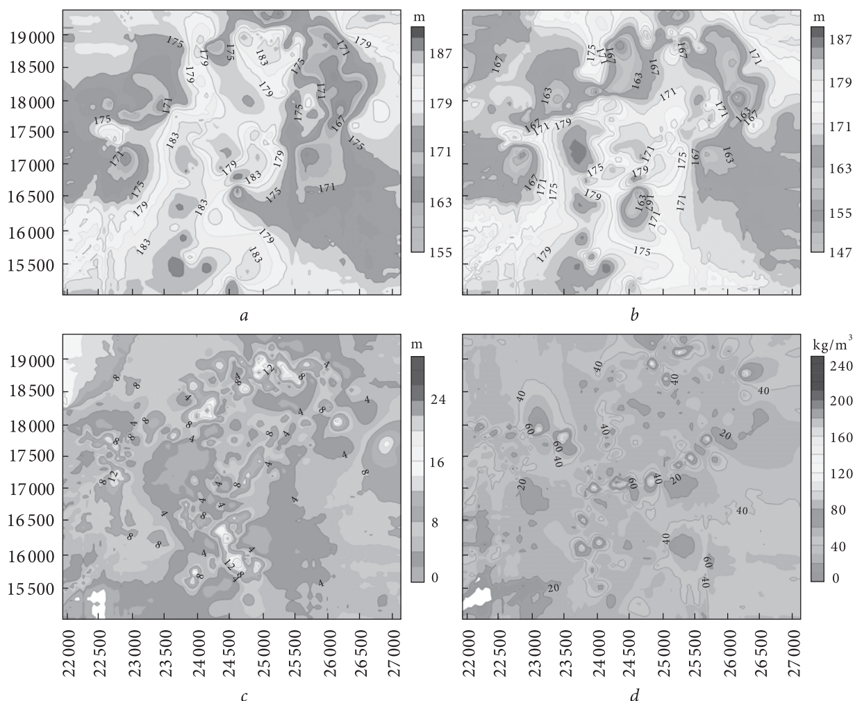
Рис. 4. Ізогіпси покрівлі (а), підшови (b), ізопахіти товщини (с) кори вивітрювання кристалічних порід фундаменту та латеральний розподіл середнього вмісту ільменіту в елювії (d). За даними детальної геологічної розвідки
