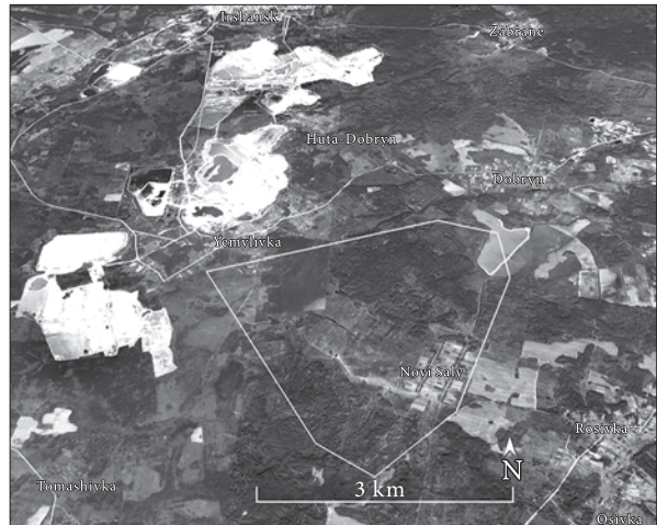
Рис. 1. Карта розміщення Тростяницького родовища на космоснімку з порталу Google Earth Pro
