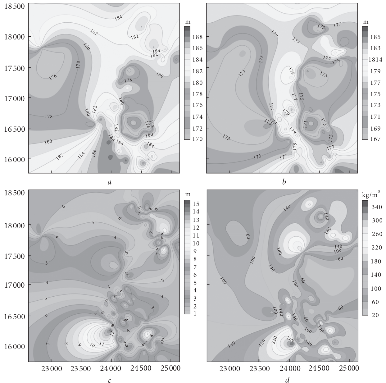
Рис. 6. Ізогіпси покрівлі (а), підшви (b), ізопакіти товщини (с) середньоярсько-нижньокрейдових алювіальних відкладів та латеральний розподіл середнього вмісту ільменіту в алювії (d). За даними попередньої геологічної розвідки
