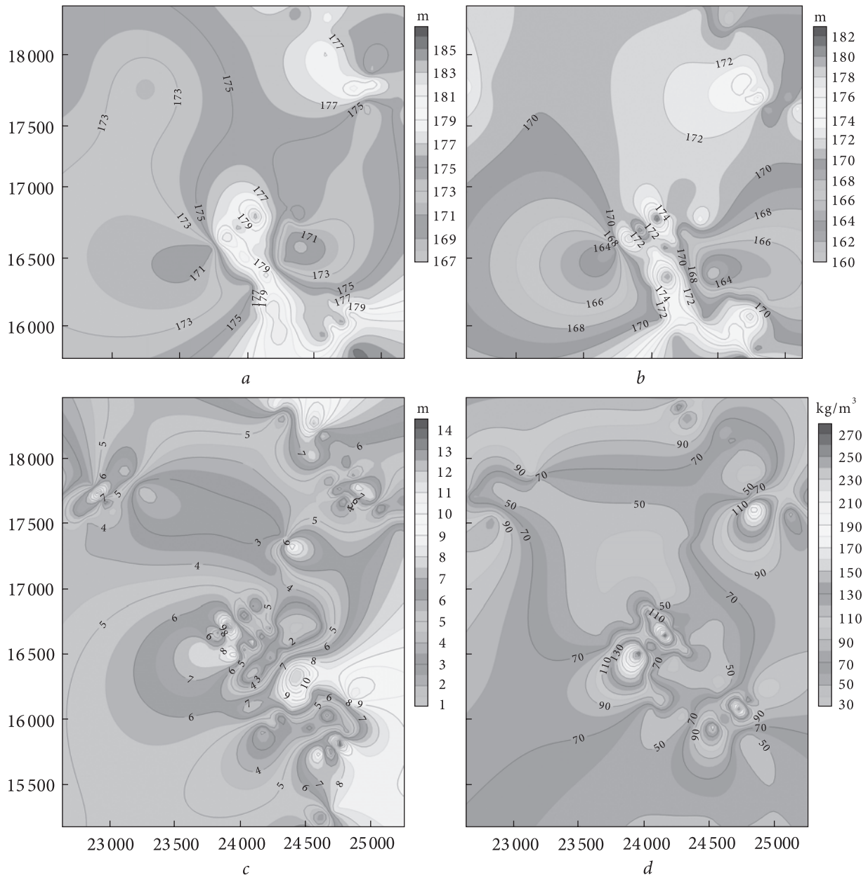
Рис. 3. Ізогіпси покрівлі (а), підшви (b), ізопахіти товщини (с) кори вивітрювання кристалічних порід фундаменту та латеральний розподіл середнього вмісту ільменіту в елювії (d). За даними попередньої геологічної розвідки
