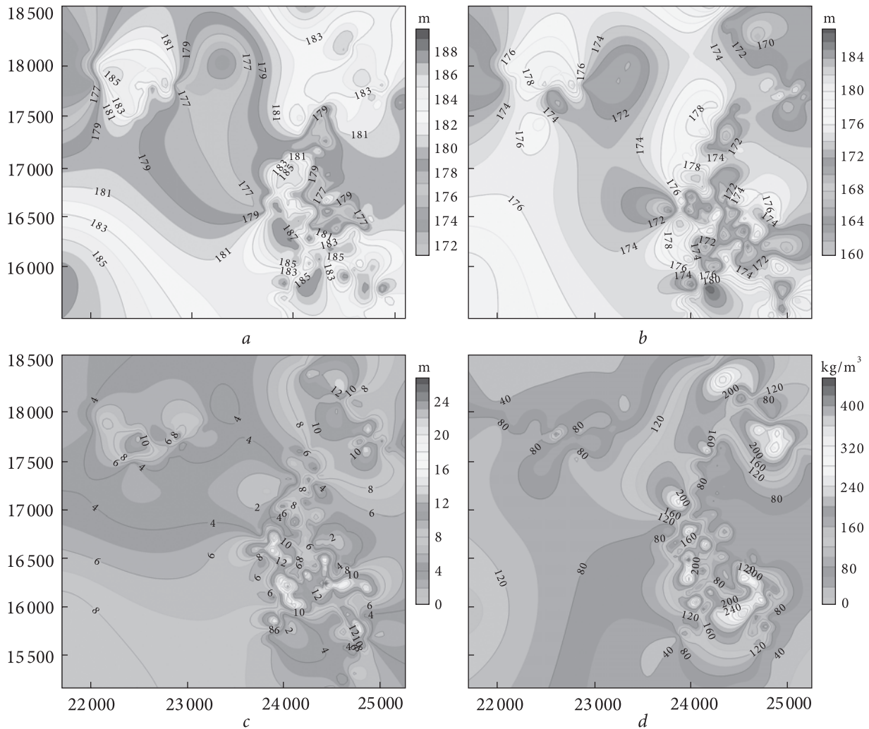
Рис. 8. Ізогіпси покрівлі (а), підшови (b), ізопахіти товщини (с) кори вивітрювання кристалічних порід фундаменту разом з середньоярсько-нижньокрейдовими алювіальними відкладами та латеральний розподіл у цій товщі порід середнього вмісту ільменіту (d). За даними попередньої геологічної розвідки
