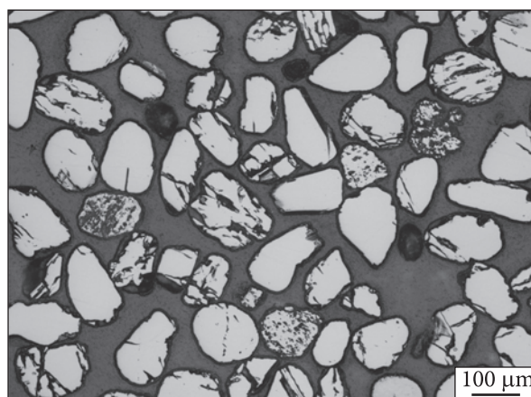
Рис. 5. Зерна рутилу Вовчанського циркон-рутил-ільменітового родовища (мікроскоп Nikon Eclipse LV100POL, зб. 10)
