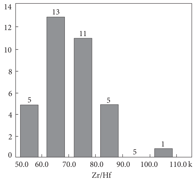
Рис. 10. Гістограми вмісту HfO 2 і співвідношення Zr/Hf в цирконах Вовчанського родовища
