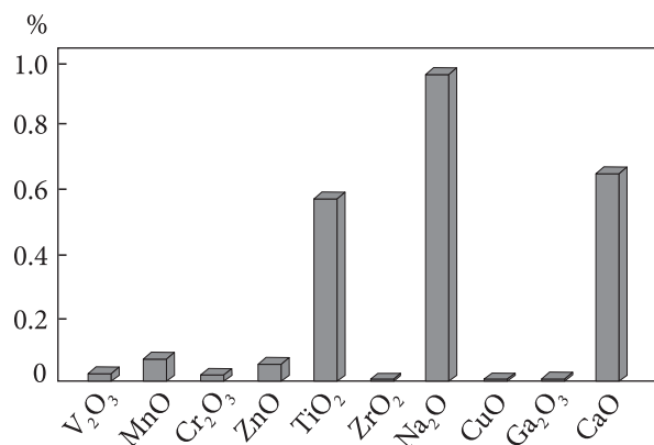
Рис. 14. Вміст домішок у ставроліті Вовчанського родовища
