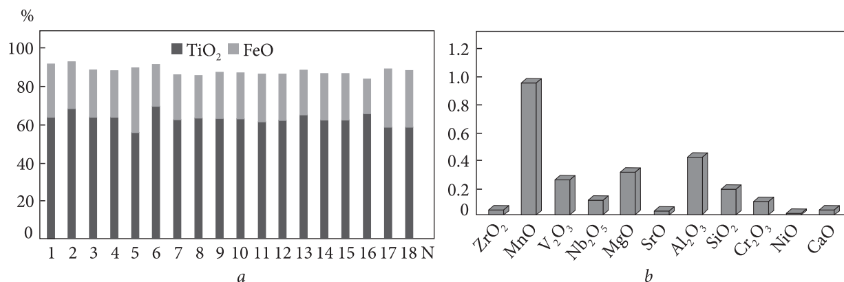
Рис. 4. Вміст \text{TiO}_2 і \text{FeO} (a) та домішок (b) в ільменіті Вовчанського родовища Fig. 4. Content of \text{TiO}_2 and \text{FeO} (a) and impurities (b) in ilmenite of the Vovchansk deposit
