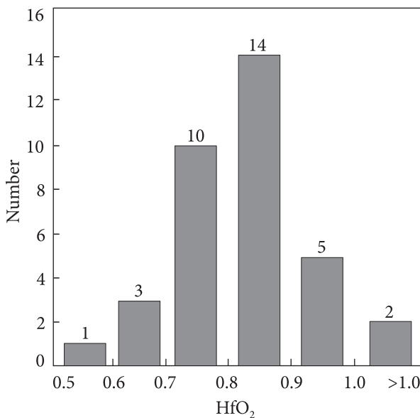
Рис. 10. Гістограми вмісту HfO 2 і співвідношення Zr/Hf в цирконах Вовчанського родовища
