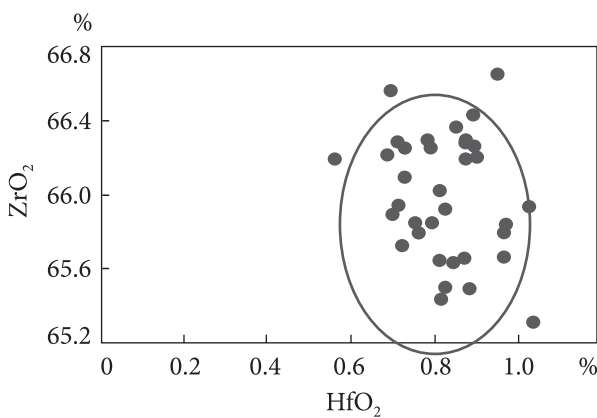
Рис. 9. Розподіл цирконів Вовчанського родовища відповідно до вмісту ZrO 2 і HfO 2
