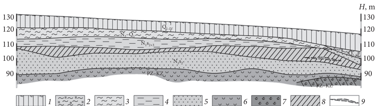
Рис. 2. Геологічний розріз Вовчанського родовища: 1 — ґрунтово-рослинний шар. Суглинки палево-жовті та жовто-бурі (четвертинна система); 2 — суглинки та глини червоно-бурі, перевідкладені (алювіальні) (четвертинна система); 3 — глини червонувато-бурі, щільні, вапнякові (плейстоцен); 4 — глини зеленувато-сірі, місцями строкаті, пластичні (верхній міоцен); 5 — піски кварцові, дрібнозернисті (олігоцен, міоцен); 6 — каолін білий, первинний, місцями строкатий (палеозой-кайнозой); 7 — вивітрені та сильно вивітрені породи основного та кислого складу (палеозой-кайнозой); 8 — рудне тіло; 9 — прошарки пісків із вмістом ільменіту нижче кондиції
