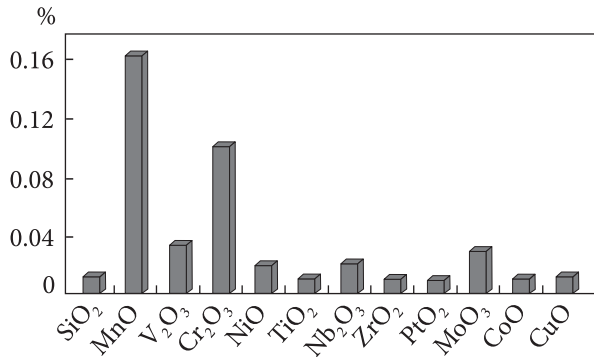
Рис. 16. Вміст домішок у ганіті Вовчанського родовища
