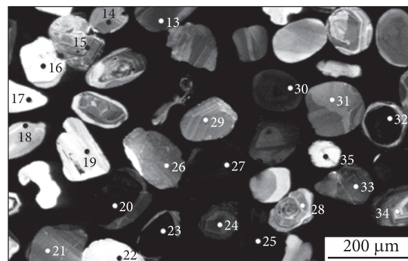
Рис. 7. BS-фото зразка цирконів Вовчанського родовища з точками аналізу
