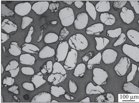
Рис. 3. Зерна ільменіту Вовчанського циркон-рутил-ільменітового родовища (мікроскоп Nikon Eclipse LV100POL , зб. 10)
