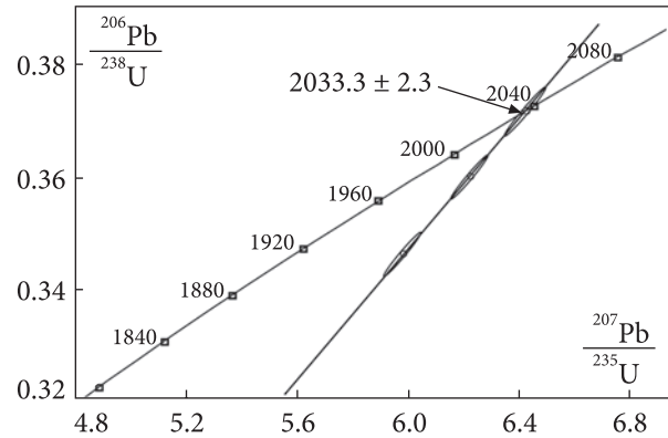
Рис. 6. Уран-свинцева діаграма з конкордією для мультизернових наважок монациту із апліто-пегматоїдного граніту, пр. 21/23
