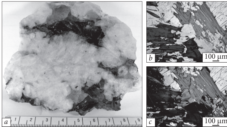
Рис. 10. Плагіопегматит, пр. 23/23: a — загальний вигляд пегматиту; b — виокремлення біотиту в плагіопегматиті. Оптичний мікроскоп Carl Zeiss Axio Imager 2 for materials, без аналізатора; c — те саме, аналізатор уведений
