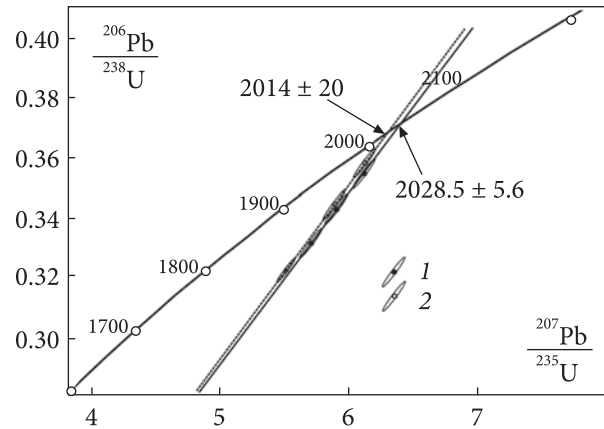
Рис. 12. Уран-свинцева діаграма з конкордією для мультизернових наважок монацитів із плагіопегматиту, пр. 23/23
