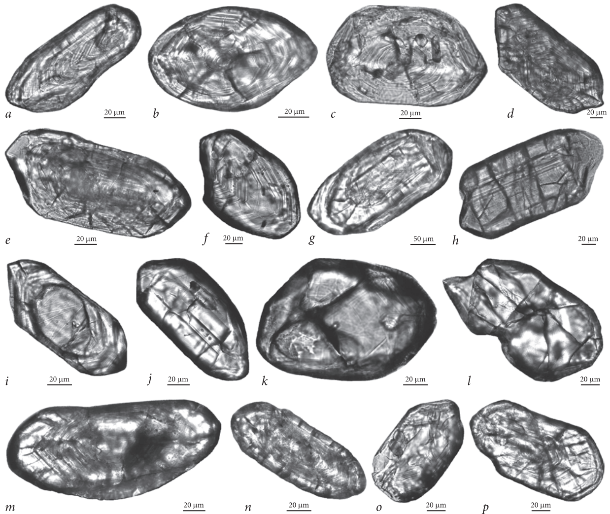
Рис. 9. Мікрофотографії зрізів кристалів циркону із гнейсу, пр. 22/23. Оптичний мікроскоп Carl Zeiss Axio Imager 2 for materials, без аналізатора. Пояснення у тексті
