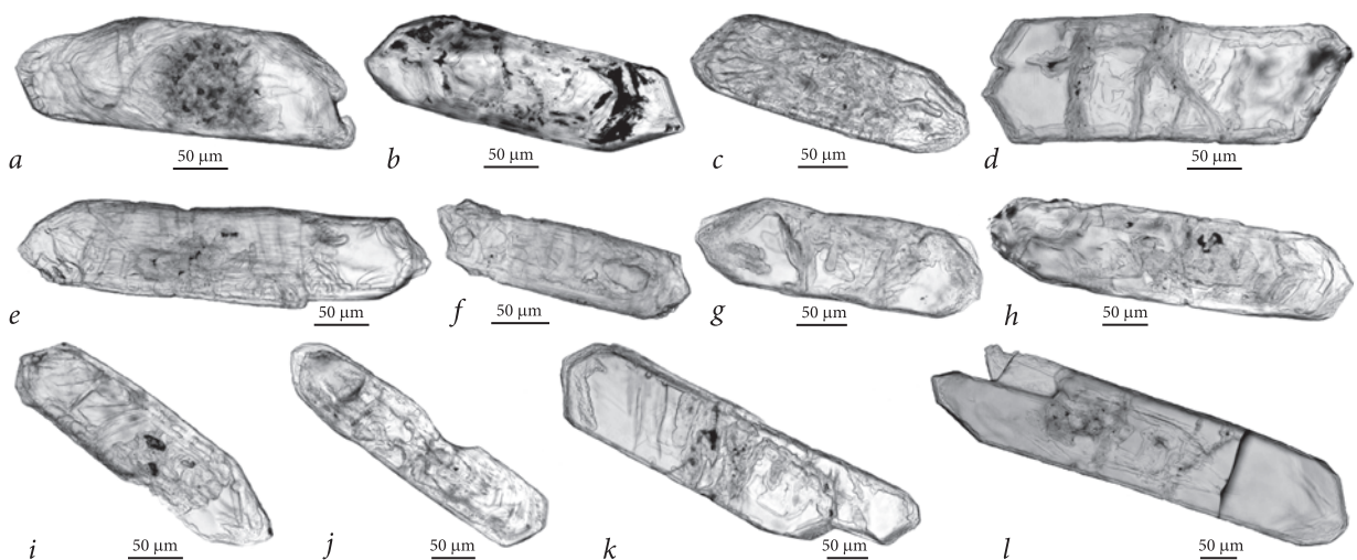
Рис. 11. Мікрофотографії зрізів кристалів циркону із пегматиту, пр. 23/23. Оптичний мікроскоп Carl Zeiss Axio Imager 2 for materials, без аналізатора. Пояснення у тексті
