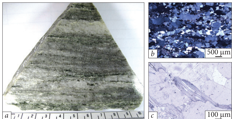
Рис. 7. Гнейс, пр. 22/23: а — загальний вигляд гнейсу; b — гранобластова структура граніту, оптичний мікроскоп Carl Zeiss Axio Imager 2 for materials, аналізатор введений; c — хлоритизований біотит, те саме, без аналізатора
