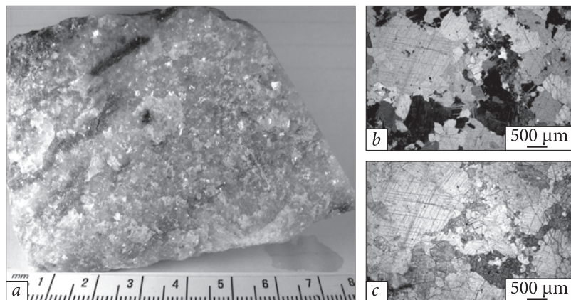
Рис. 13. Кальцифір, пр. 24/23: a — загальний вигляд; b — повнокристалічна гранобластова структура кальцифіру з елементами тектонобластезу, оптичний мікроскоп Carl Zeiss Axio Imager 2 for materials, з аналізатором; c — те саме, без аналізатора
