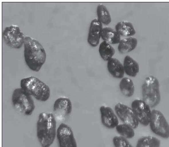
Рис. 8. Мікрофотографія кристалів циркону із гнейсу, пр. 22/23. Бінокулярний мікроскоп SZM-45T2
