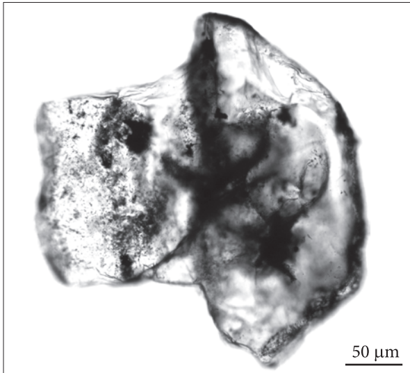
Рис. 5. Мікрофотографія світло-коричневого напівпрозорого кристала монациту, граніт апліто-пегматоїдний, пр. 21/23. Оптичний мікроскоп Carl Zeiss Axio Imager 2 for materials, без аналізатора
