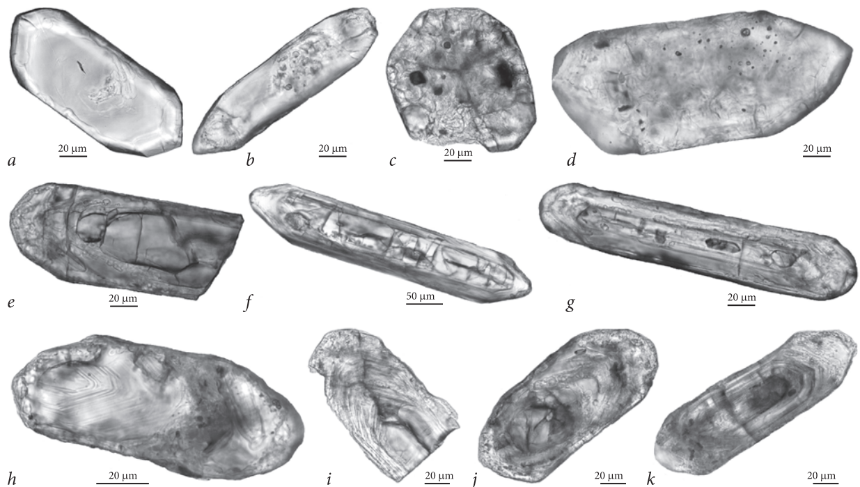
Рис. 4. Мікрофотографії зрізів кристалів циркону із апліто-пегматоїдного граніту, пр. 21/23, оптичний мікроскоп Carl Zeiss Axio Imager 2 for materials, без аналізатора. Пояснення у тексті
