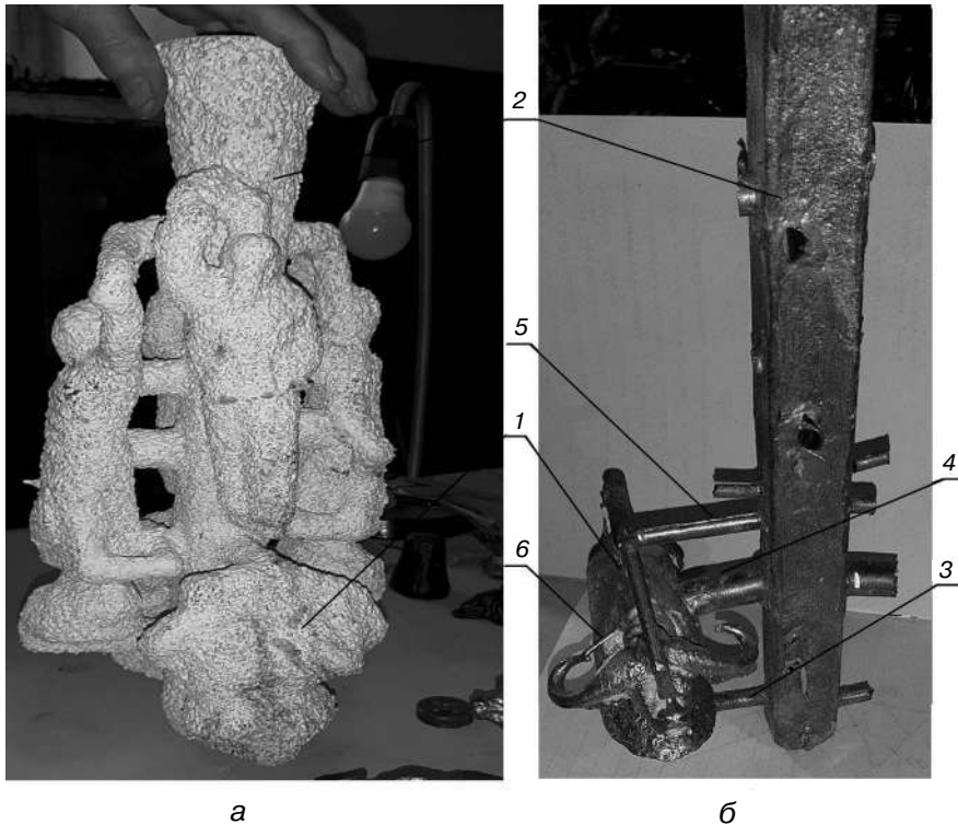
Рис. 2. Загальний вигляд форми при литті по моделям, що витоплюються (а), і виливок «Буйвол» з ливниково-живильною системою (б): 1 – виливок «Буйвол»; 2 – стояк; 3 – живильник в нижню частину виливку; 4 – живильник в центральну масивну частину «Буйвола»; 5 – живильник в верхню частину виливку; 6 – живильники до рогів
