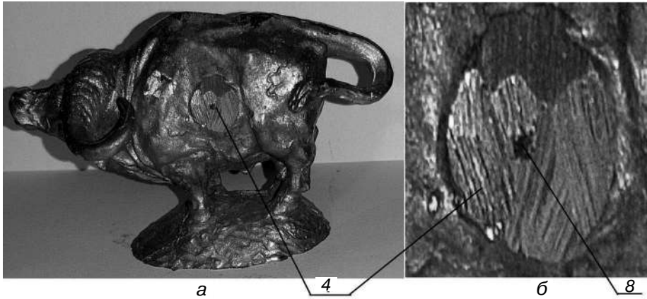
Рис. 3. «Буйвол» після видалення ливника \varnothing 12 мм (а) і збільшене зображення (б) усадочної пористості в центрі масивної частини виливку: 4 – залишки живильника до масивної частини виливка; 8 – усадочна пористість в центрі живильника
