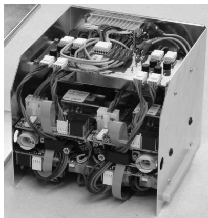
Fig. 8. LVPS Box
