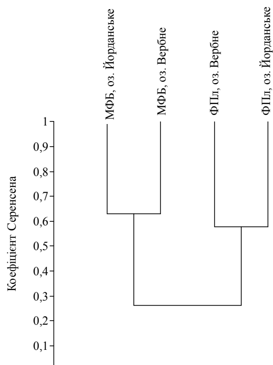
Рис. 3. Дендрограма подібності видового складу фітопланктону та мікрофітобентосу озера Вербне та Йорданське (узагальнені дані) за коефіцієнтом Серенсена
