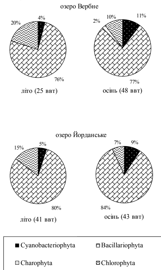
Рис. 2. Таксономічне різноманіття мікрофітобентосу озер Вербне та Йорданське
