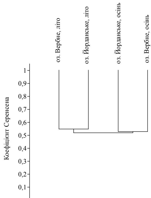
Рис. 5. Дендрограма подібності видового складу мікрофітобентосу озера Вербне і Йорданське в різні сезони за коефіцієнтом Серенсена
