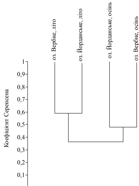
Рис. 4. Дендрограма подібності видового складу фітопланктону озера Вербне та Йорданське в різні сезони за коефіцієнтом Серенсена
