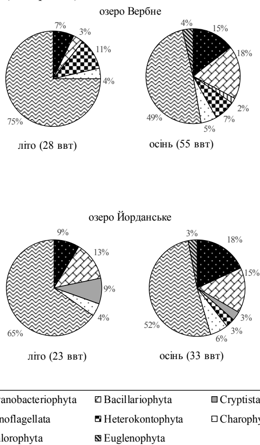
Рис. 1. Таксономічне різноманіття фітопланктону оз. Вербне та Йорданське
