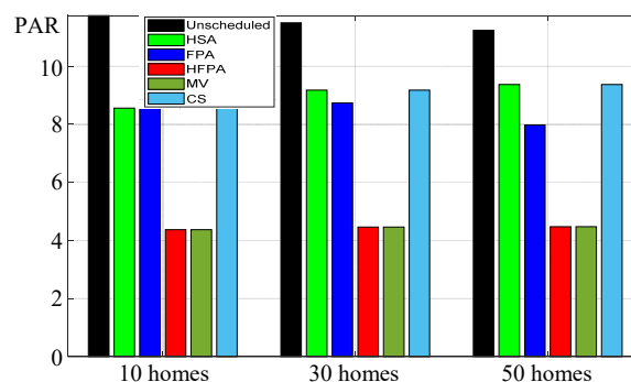
Fig. 3. PAR against different OTIs
