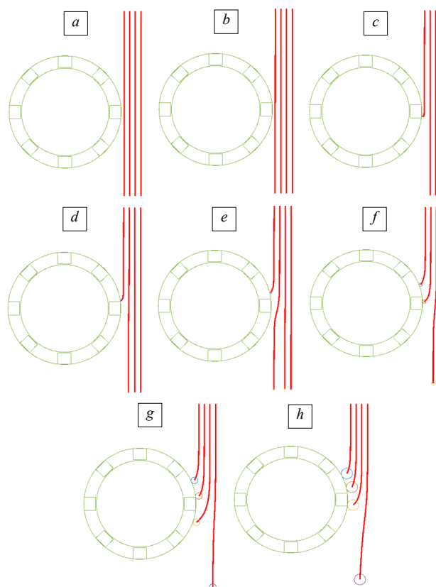
Fig. 8. Computed particle trajectories obtained in granular medium: a) D_p=70 \cdot 10^{-6} \text{ m} ; b) D_p=150 \cdot 10^{-6} \text{ m} ; c) D_p=300 \cdot 10^{-6} \text{ m} ; d) D_p=800 \cdot 10^{-6} \text{ m} ; e) D_p=1500 \cdot 10^{-6} \text{ m} ; f) D_p=3000 \cdot 10^{-6} \text{ m} ; g) D_p=6000 \cdot 10^{-6} \text{ m} ; h) D_p=10000 \cdot 10^{-6} \text{ m}
